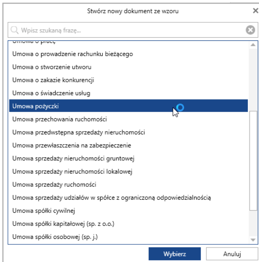
Rys. 8. Kreator dokumentu
