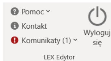
Rys. 25 Komunikaty systemowe
